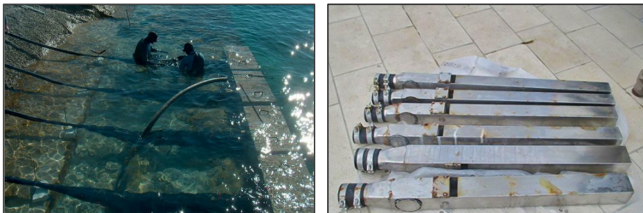
Slika 4. Dijelovi cijevnog sustava Morskih orgulja: lijevo, PE potopljene cijevi [1] i desno, inox akustične cijevi [2]
